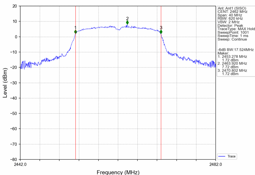
802.11n(HT20)_HCH_2462MHz_Ant1 (SISO)_NTNV
