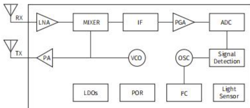
天线模块框图(Antenna module block diagram)
