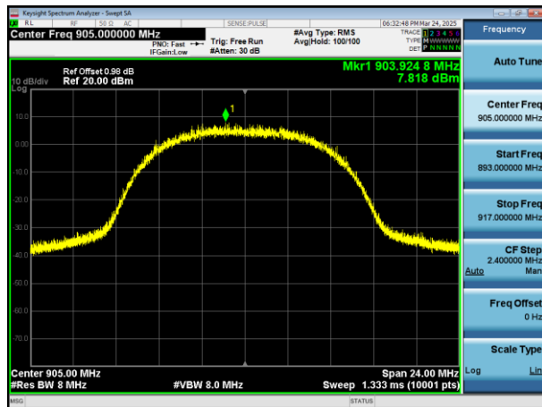
802.11ah_2M
