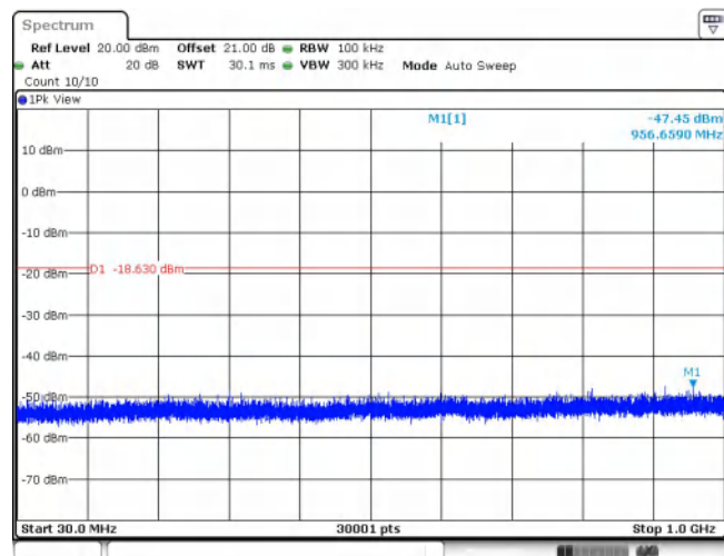
11N20MIMO_Ant2_2437_0~Reference
