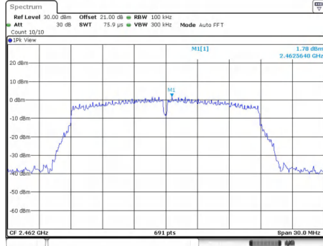
11N20MIMO_Ant2_2462_0~Reference
