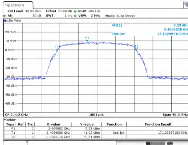
11G_Ant2_2412
