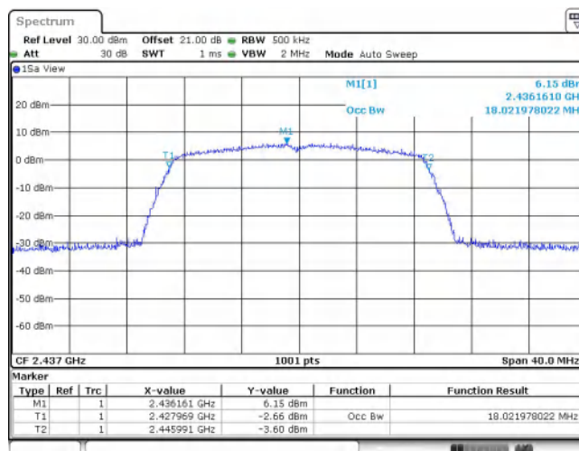
11N20MIMO_Ant1_2437
