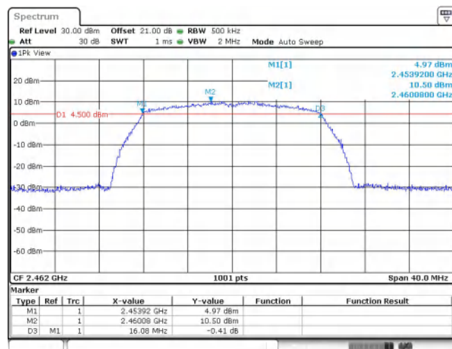
11G_Ant2_2462
