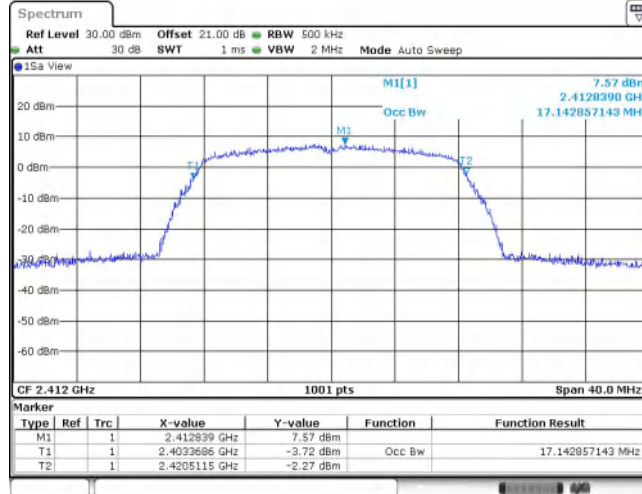
11G_Ant1_2412
