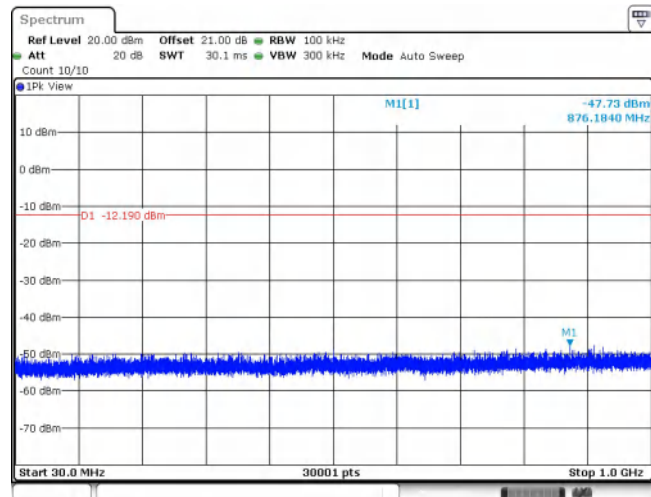
11B_Ant2_2462_30~1000
