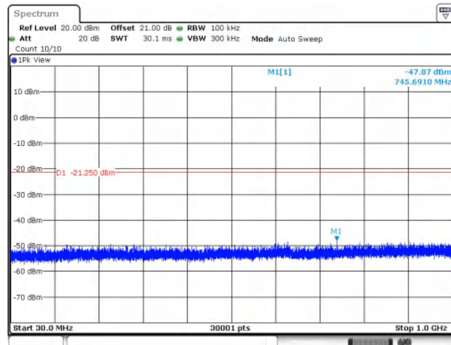
11N20MIMO_Ant1_2412_30~1000
