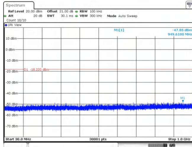
11N20MIMO_Ant2_2462_30~1000
