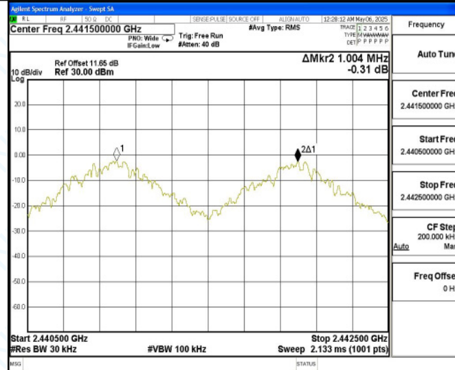
2DH5_Ant1_Hop
