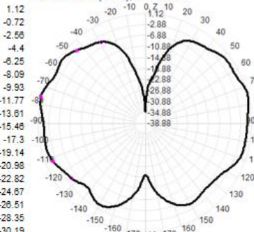
2440.0MHz Total(E1-XZ), Max= 1.12dBi
