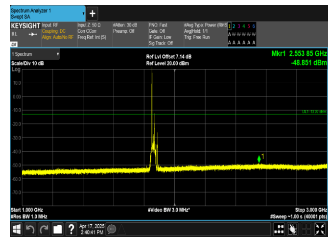
Band2-20MHz-QPSK-18700-1RB#0-1000~3000-PASS
