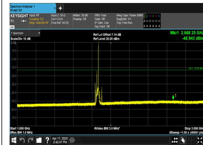
Band2-20MHz-QPSK-18700-1RB#99-1000~3000-PASS
