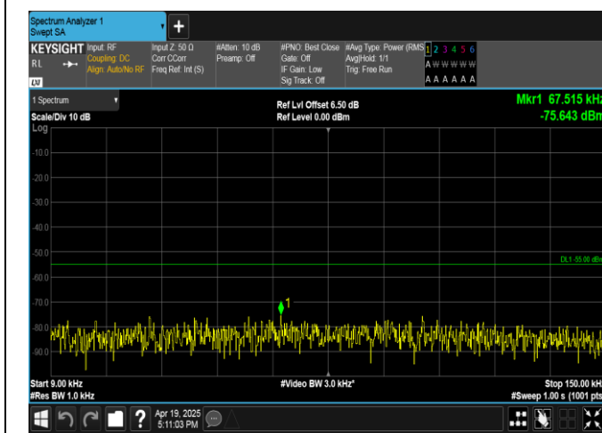
Band7-10MHz-QPSK-20800-50RB#0-0.009~0.15-PASS
