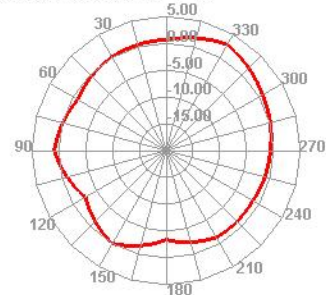
5850.000MHz E2
