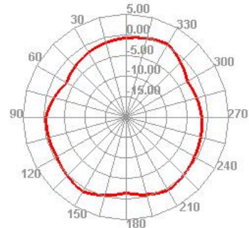
5150.000MHz E2
