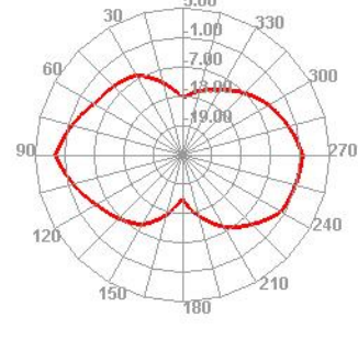
5850.000MHz H
