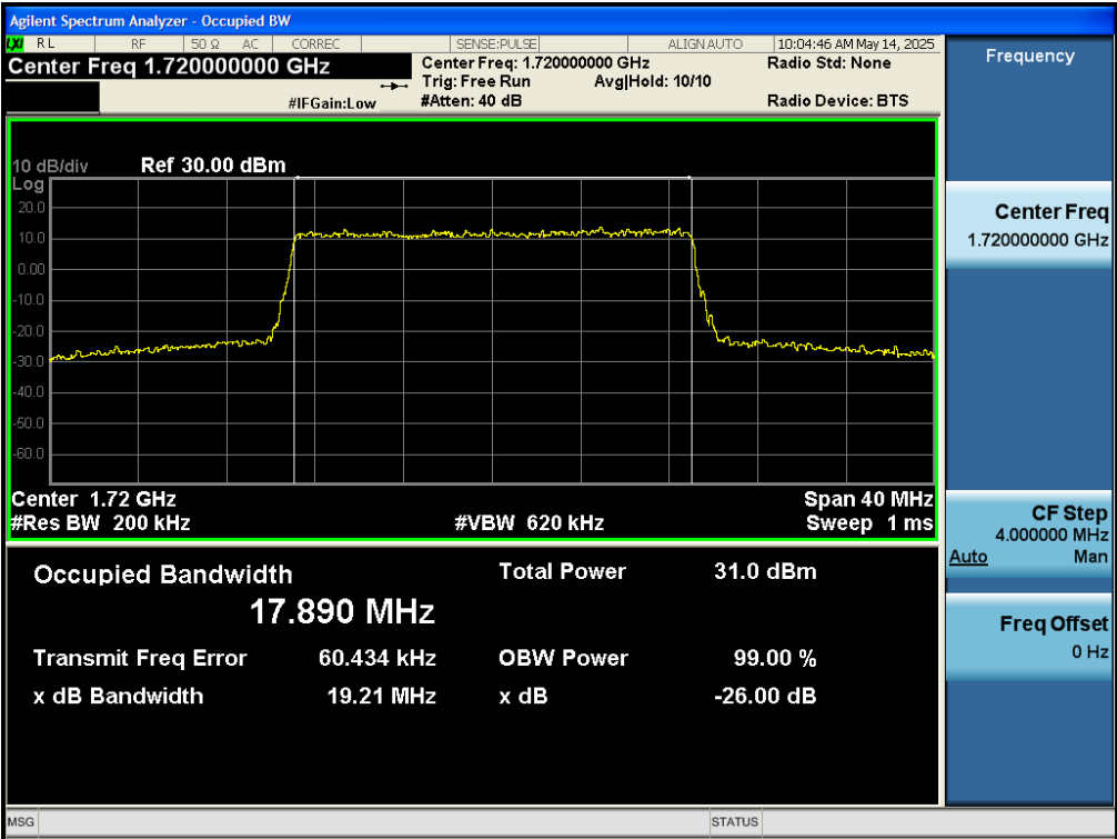
Test_Graph_band4_1720MHz_20M_QPSK_100RB#LOW_OBW&EBW
