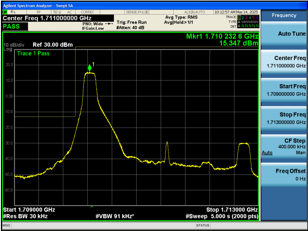
Test_Graph_band4_1711.5MHz_3M_QPSK_1RB#LOW_Band edge
