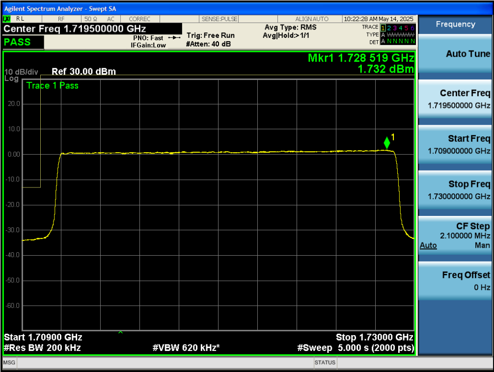
Test_Graph_band4_1720MHz_20M_16QAM_100RB#LOW_Band edge
