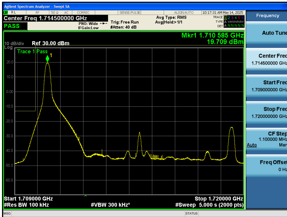
Test_Graph_band4_1715MHz_10M_QPSK_1RB#LOW_Band edge
