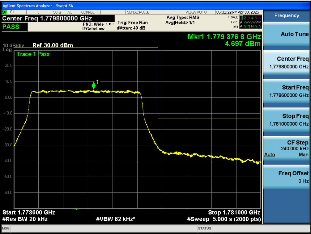
Test_Graph_band66_1779.3MHz_1.4M_16QAM_6RB#LOW_Band edge
