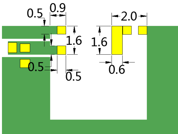
打孔参考示意图 Punch reference diagram
