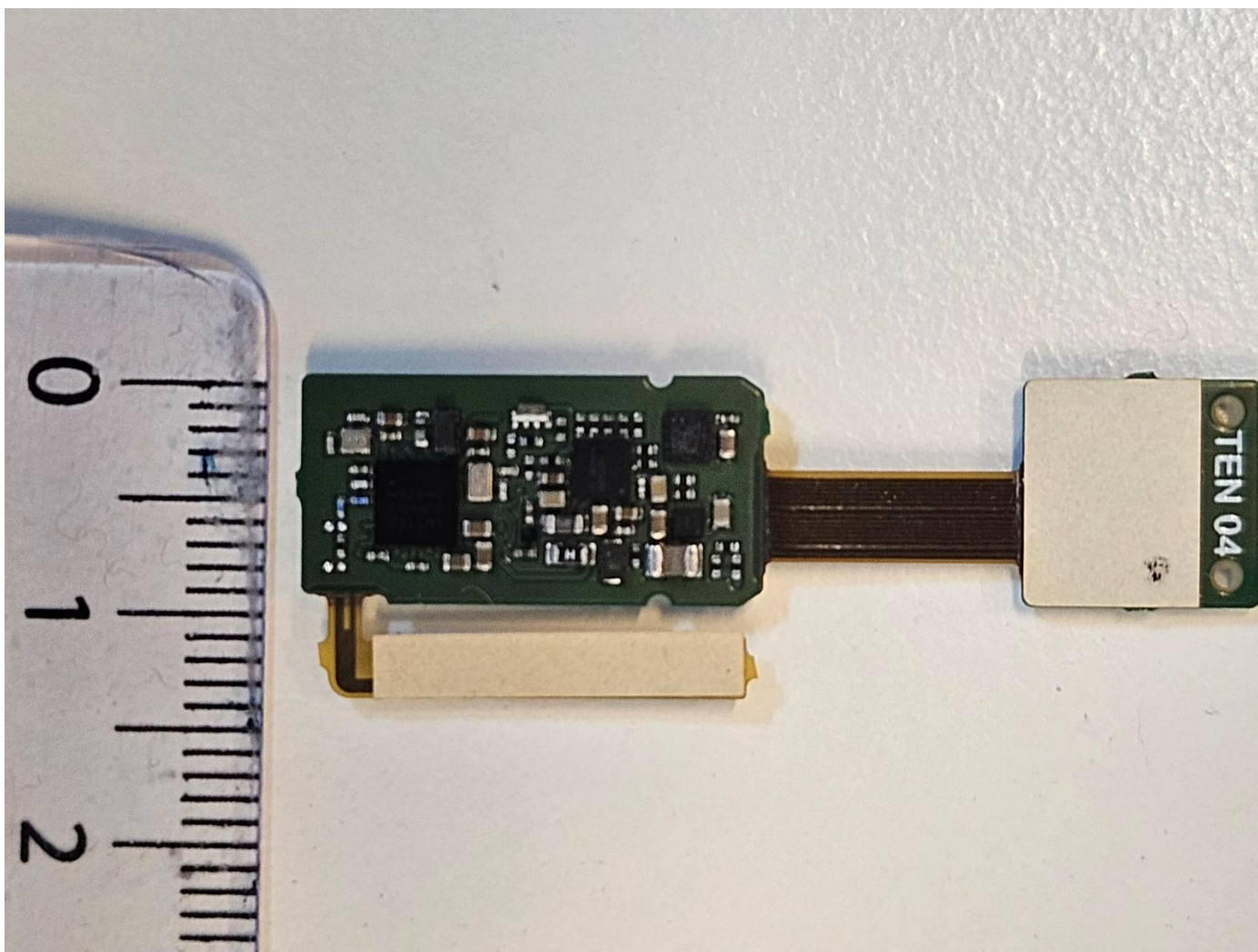
PCB bottom
