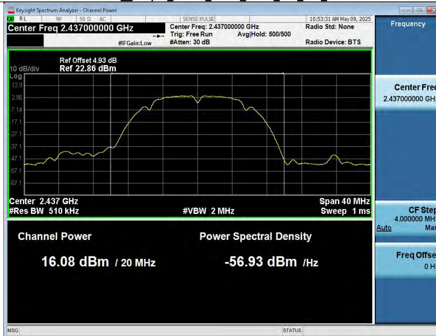
MAX_Output_Power_NVNT_ANT1_802_11b_2437
