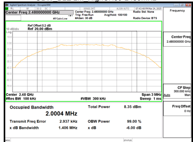
OBW BLE 2M HighCH39-2480MHz
