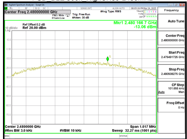
PSD BLE 500k HighCH39-2480MHz
