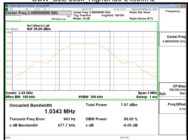
OBW BLE 500k HighCH39-2480MHz
