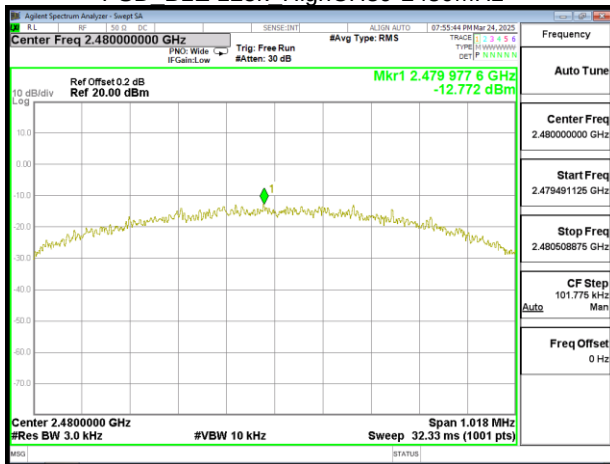
PSD BLE 125k HighCH39-2480MHz
