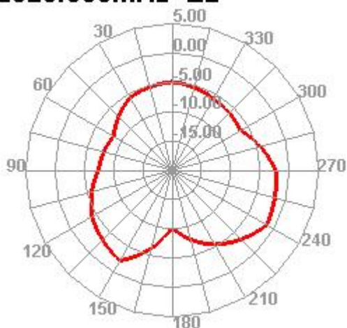
2320.000MHz E2
