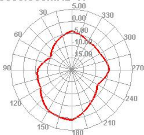
5850.000MHz H
