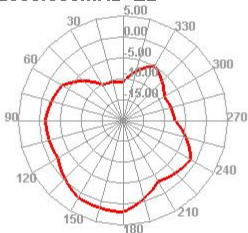
2000.000MHz E2
