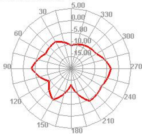
710.000MHz E2
