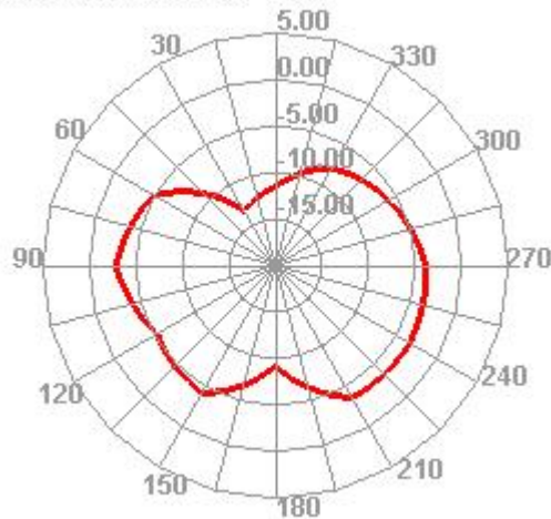
830.000MHz E2
