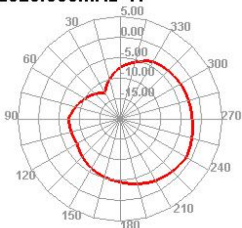
2320.000MHz H
