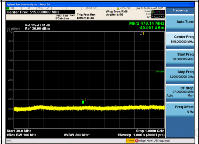
GPRS850-251-5-30~1000MHz-PASS
