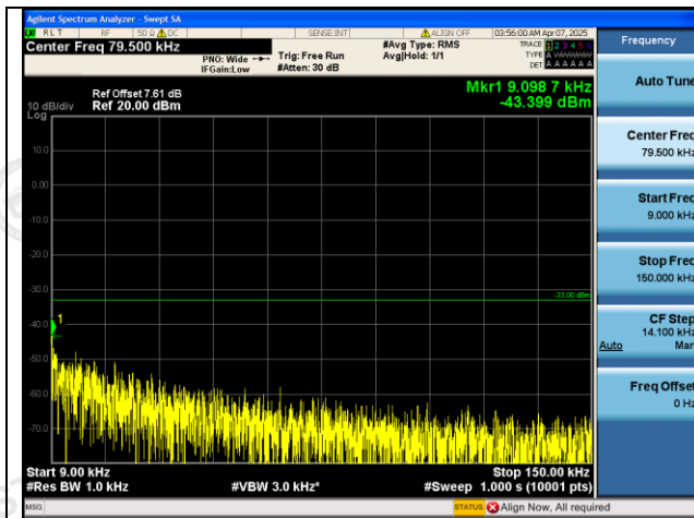
GSM850-251-5-0.009~0.15MHz-PASS
