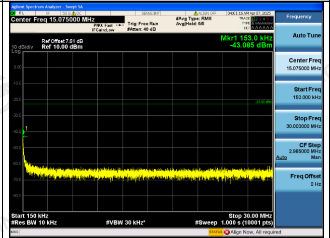
GPRS850-251-5-0.15~30MHz-PASS
