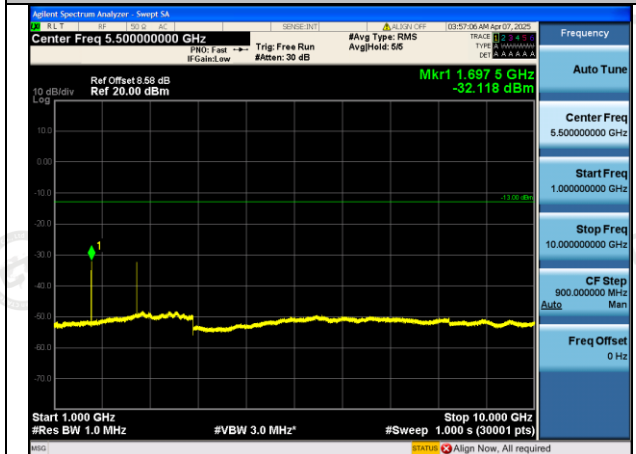
GSM850-251-5-1000~10000MHz-PASS
