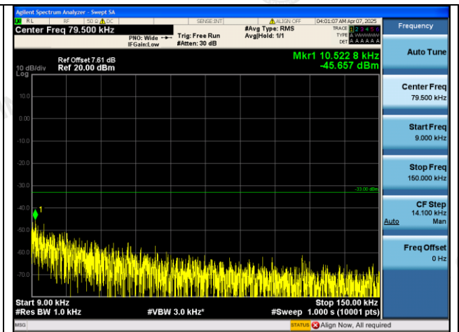
GPRS850-251-5-0.009~0.15MHz-PASS
