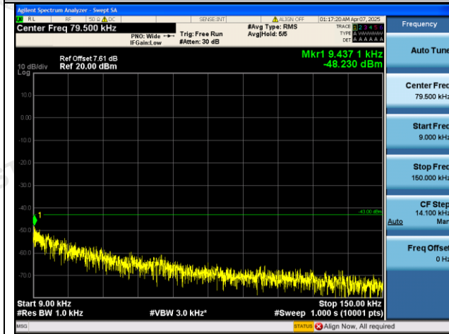
GSM1900-661-0-0.009~0.15MHz-PASS
