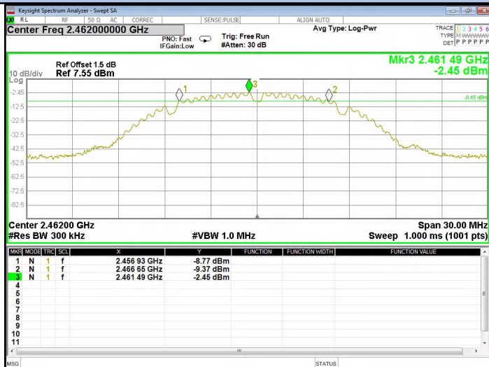
IEEE 802.11b_Ant1_CH11 2462MHz
