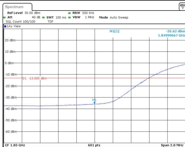
Band2-20MHz-16QAM-19100-1RB#0
