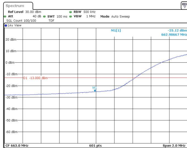
Band71-20MHz-QPSK-133372-1RB#0
