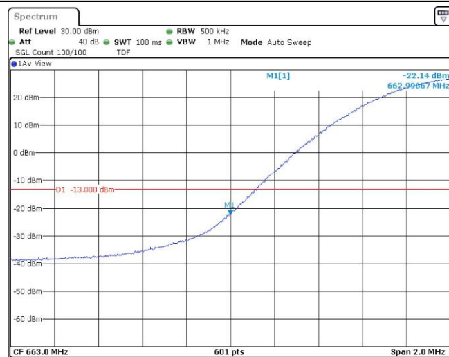
Band71-20MHz-QPSK-133222-1RB#99
