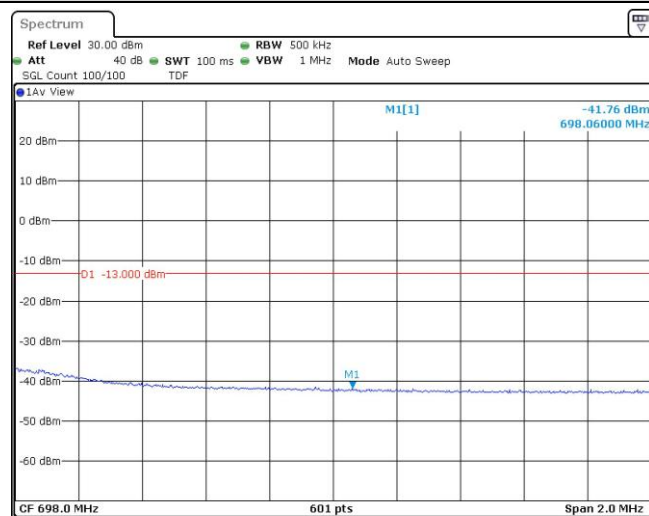
Band71-20MHz-QPSK-133372-1RB#99
