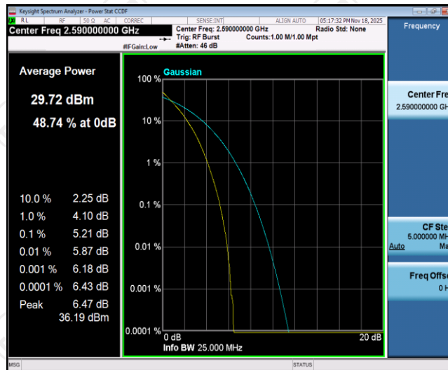
Band41-20MHz-QPSK-40590-100RB#0
