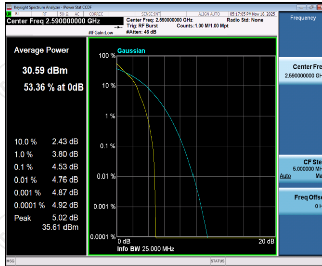
Band41-20MHz-QPSK-40590-1RB#0
