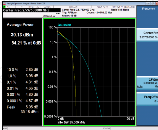
Band41-5MHz-QPSK-40065-1RB#0
