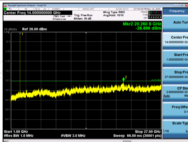
Band41-5MHz-QPSK-40590-1RB#0-Range2:1000~27000MHz
