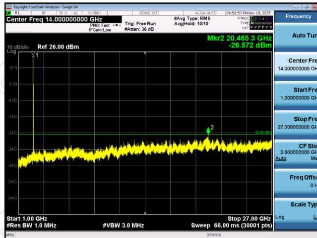
Band41-5MHz-QPSK-40065-1RB#0-Range2:1000~27000MHz
