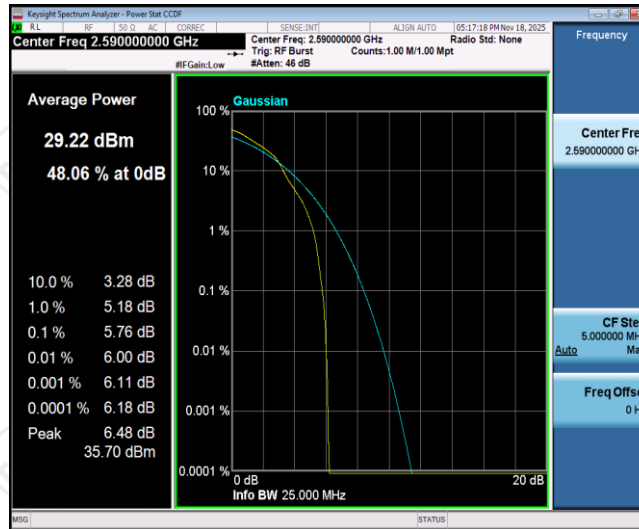
Band41-20MHz-16QAM-40590-1RB#0
