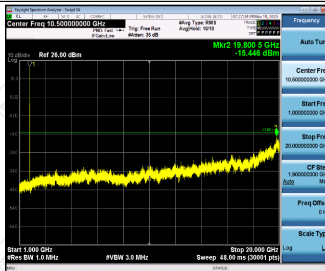
Band66-10MHz-QPSK-132622-1RB#0-Range2:1000~20000MHz
