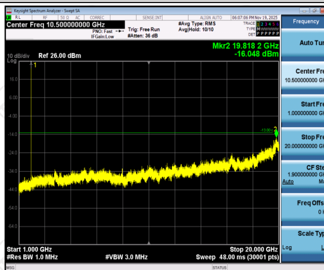
Band2-3MHz-QPSK-19185-1RB#0-Range2:1000~20000MHz
