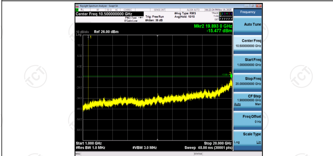
Band4-1.4MHz-QPSK-19957-1RB#0-Range2:1000~20000MHz
