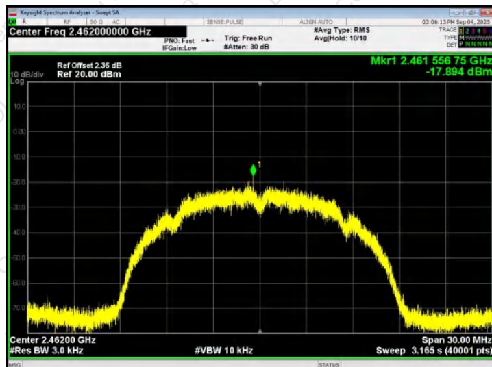
802.11b - CH11
