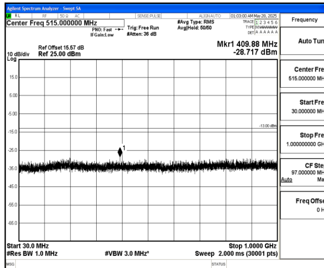
Band4-3MHz-QPSK-20175-1-0-Low-30-1000--28.72-PASS
