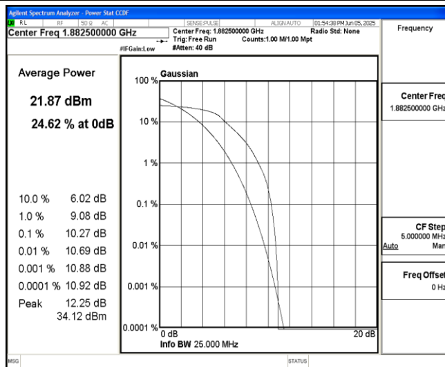
Band25-1.4MHz-QPSK-26365-6-0-Low-10.27-&lt;=13-PASS
