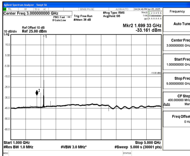
Band25-10MHz-QPSK-26365-1-0-Low-1000-5000--33.16-PASS
