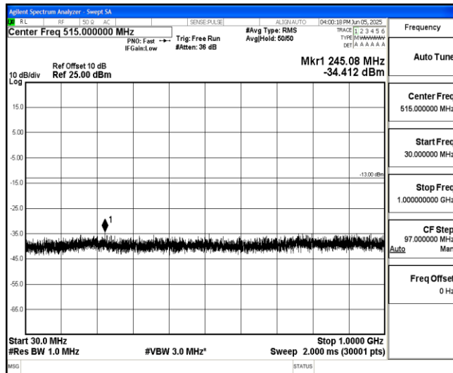
Band25-10MHz-QPSK-26090-1-0-Low-30-1000--34.41-PASS
