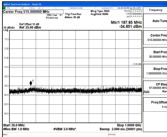
Band25-20MHz-16QAM-26140-1-0-Low-30-1000--34.85-PASS
