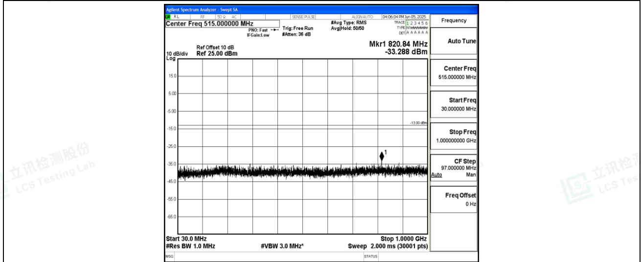
Band25-10MHz-16QAM-26365-1-0-Low-30-1000--33.29-PASS
