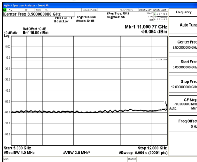
Band25-10MHz-QPSK-26365-1-0-Low-5000-12000--56.09-PASS
