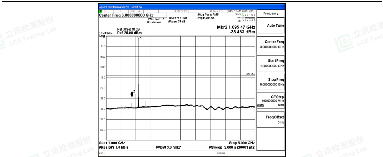
Band25-20MHz-16QAM-26365-1-0-Low-1000-5000--33.46-PASS
