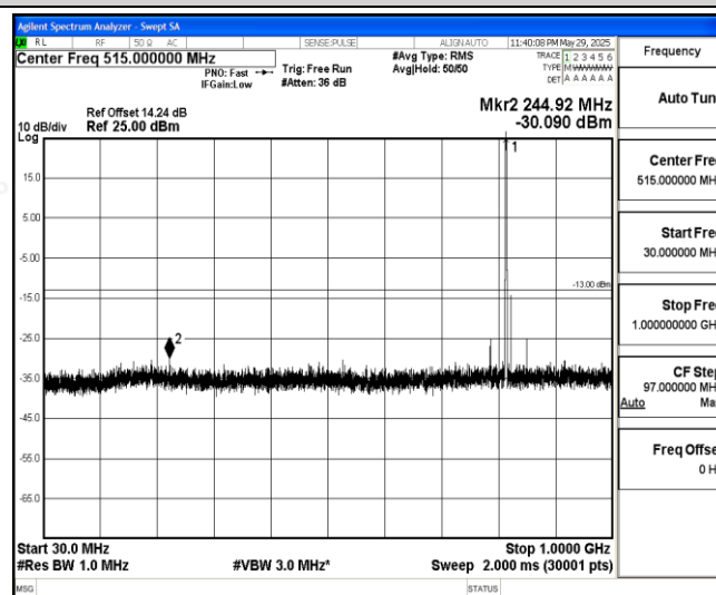
Band26-3MHz-QPSK-26740-1-0-Low-30-1000--30.09-PASS
