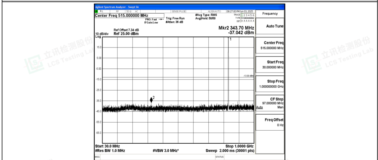
Band26-5MHz-QPSK-26915-1-0-Low-30-1000--37.04-PASS
