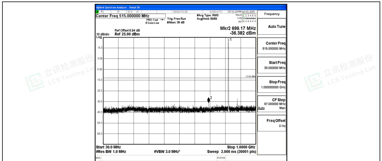
Band26-1.4MHz-QPSK-26797-1-0-Low-30-1000--36.38-PASS
