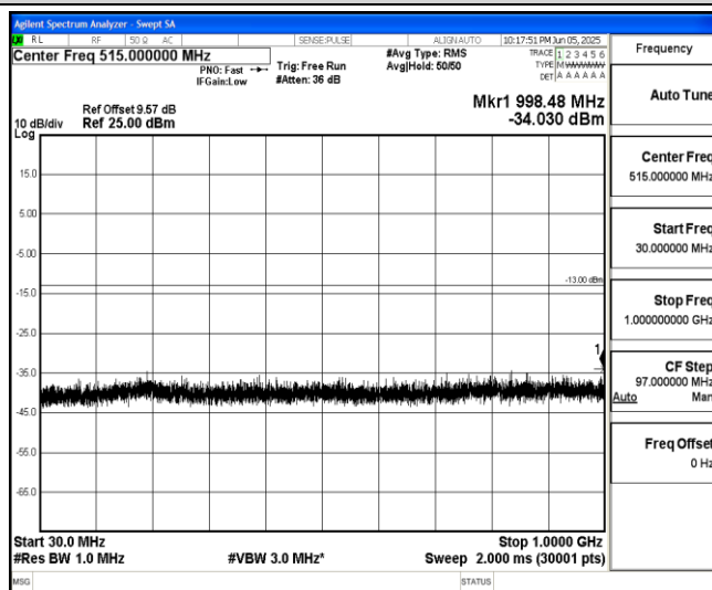
Band66-20MHz-QPSK-132322-1-0-Low-30-1000--34.03-PASS
