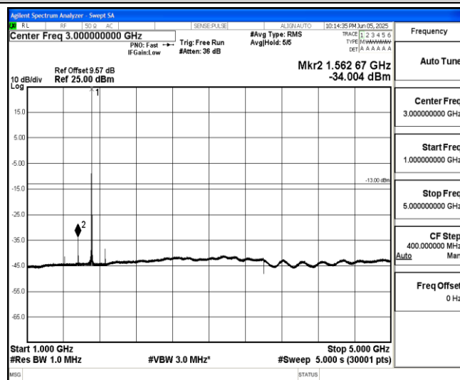
Band66-20MHz-QPSK-132072-1-0-Low-1000-5000--34-PASS
