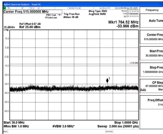
Band66-20MHz-QPSK-132072-1-0-Low-30-1000--33.97-PASS
