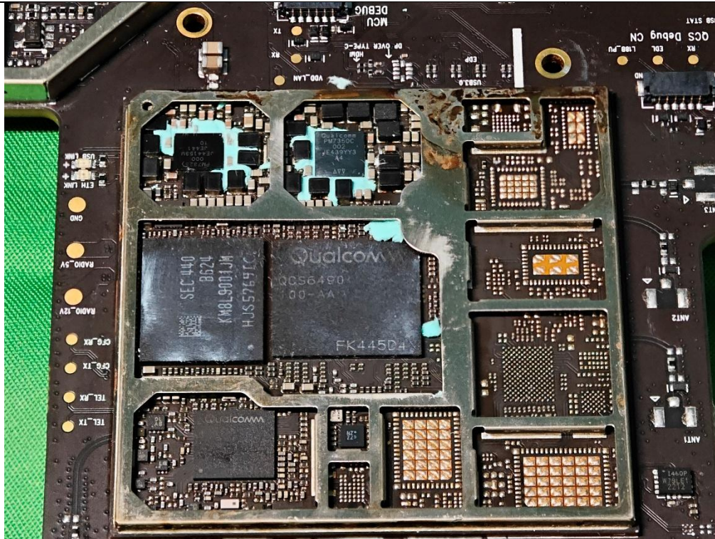
EUT Photo(8) Wi-Fi Module
