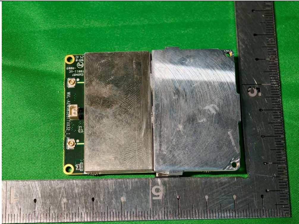
EUT Photo(12) SRD Module
