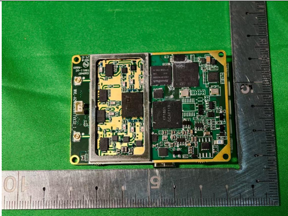
EUT Photo(14) SRD Module
