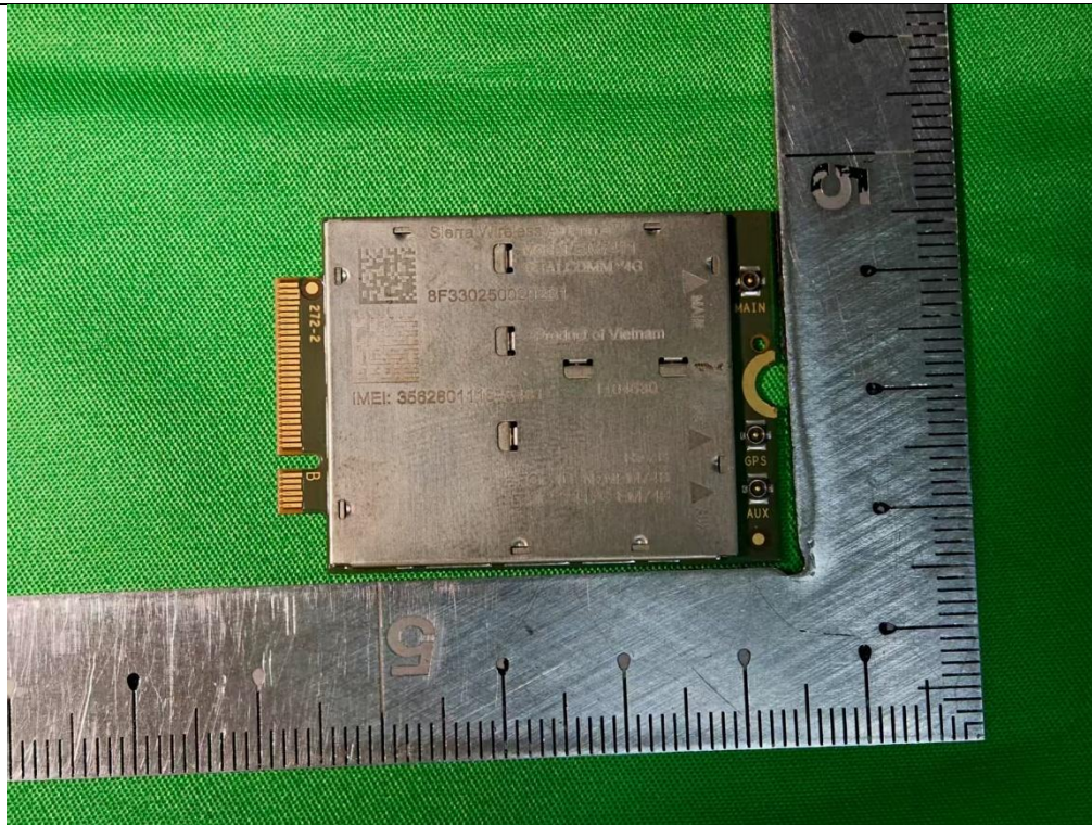
EUT Photo(10) WWAN Module
