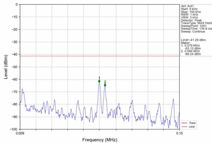
2M_MCH_2440MHz_Ant1_NTNV
