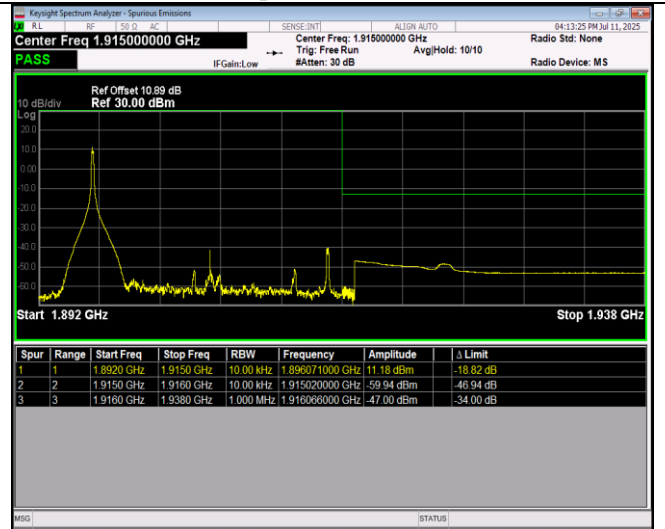
Band25-20MHz-QPSK-26590-100RB#0
