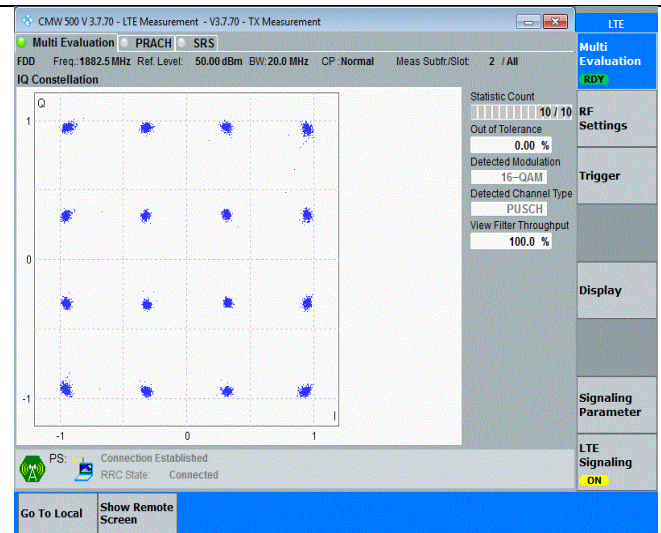
Band25-20MHz-16QAM-26365-100RB#0
