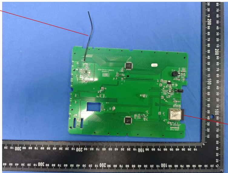
BT/WIFI ANT
