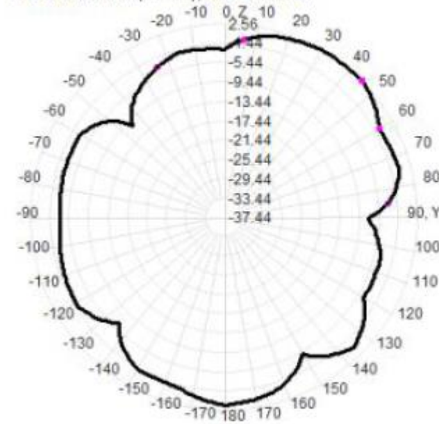
2450.0MHz Total(E2-YZ), Max= 2.56dBi
