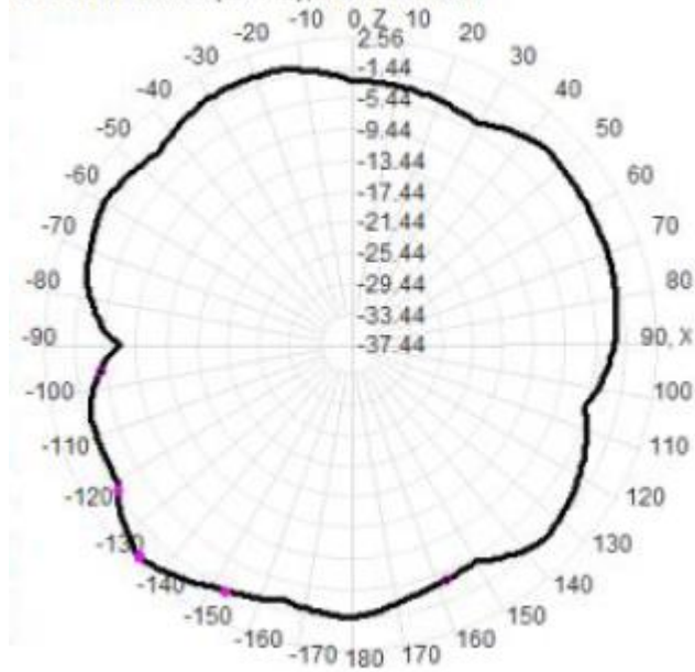
2450.0MHz Total(E1-XZ), Max= 1.54dBi
