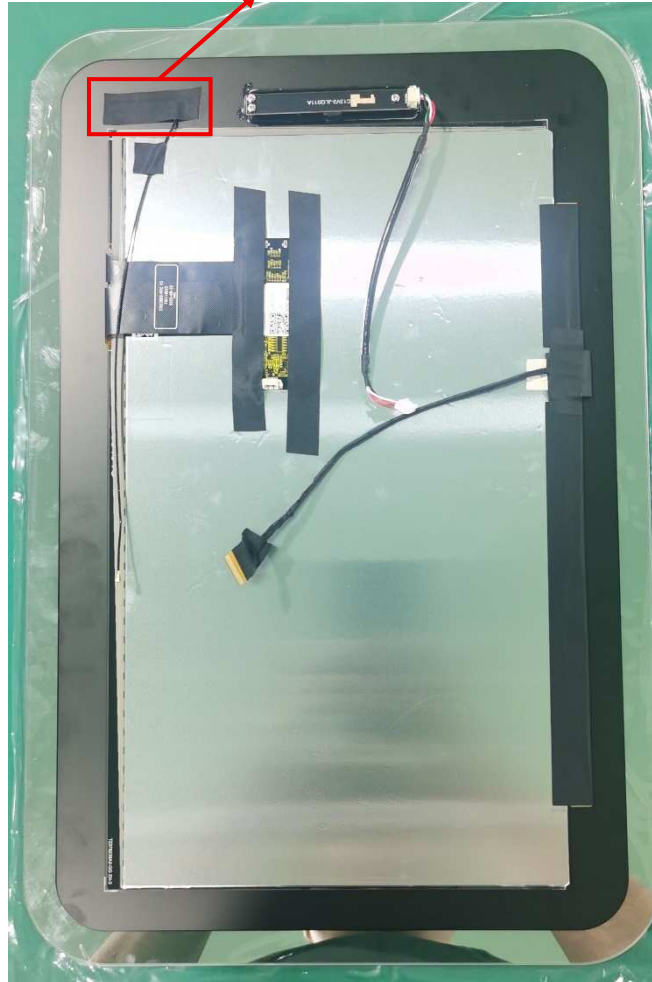
BT/WIFI Antenna
