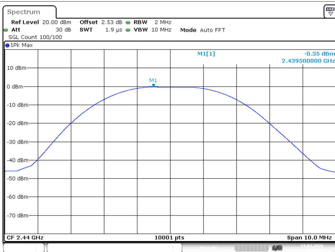
Peak Power NVNT BLE 2M 2440MHz Ant1
