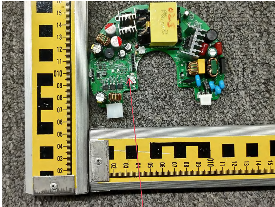
433 module
