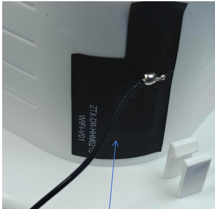
Antenna
