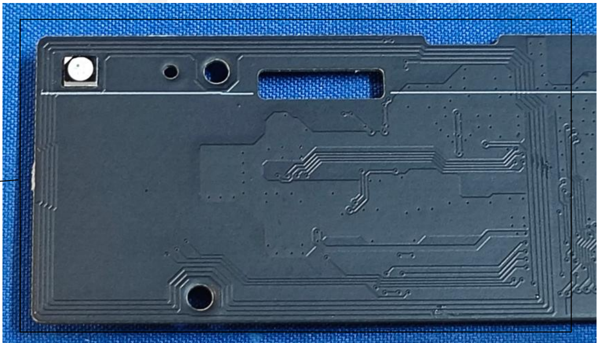
NFC antenna
