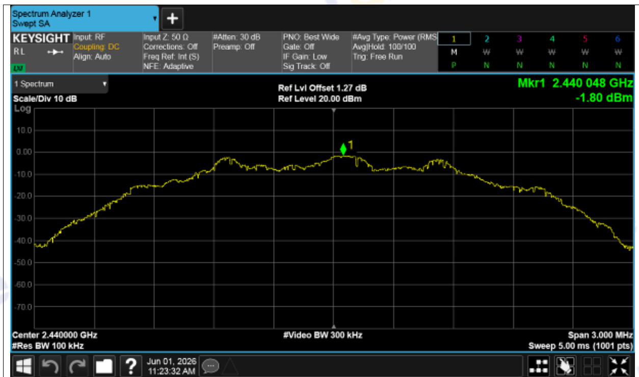
Tx. Spurious NVNT BLE 2M 2440MHz Ant1 Emission
