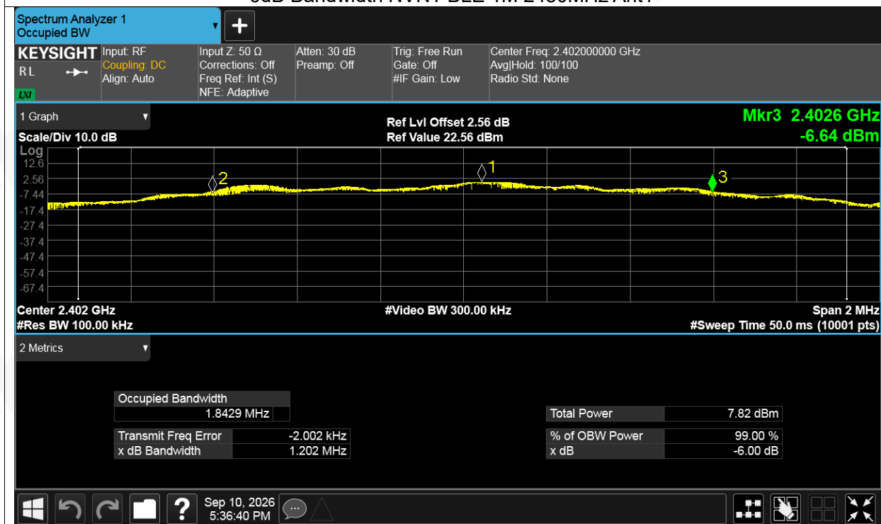
-6dB Bandwidth NVNT BLE 2M 2402MHz Ant1
