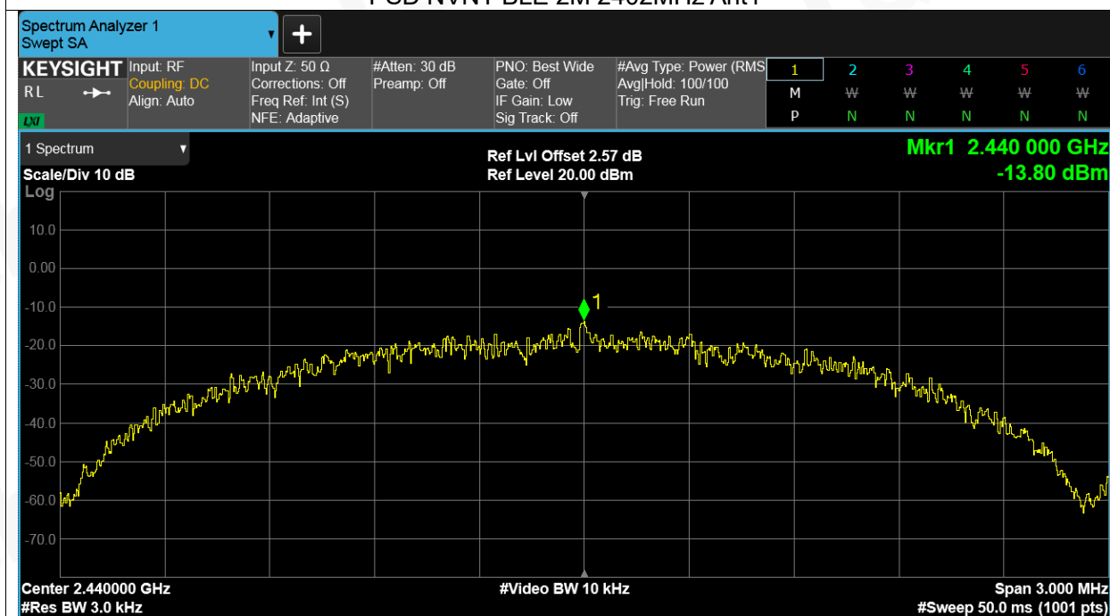
PSD NVNT BLE 2M 2440MHz Ant1
