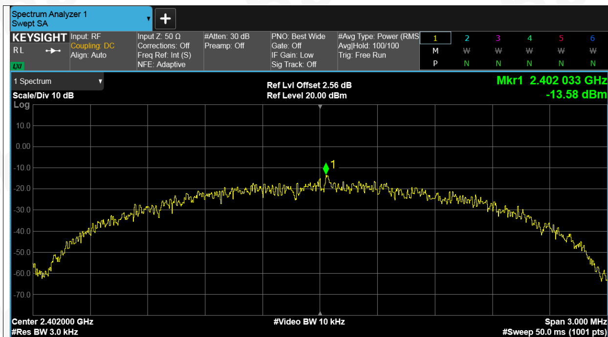
PSD NVNT BLE 2M 2402MHz Ant1
