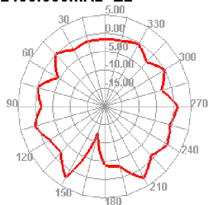
2400.000MHz E2
