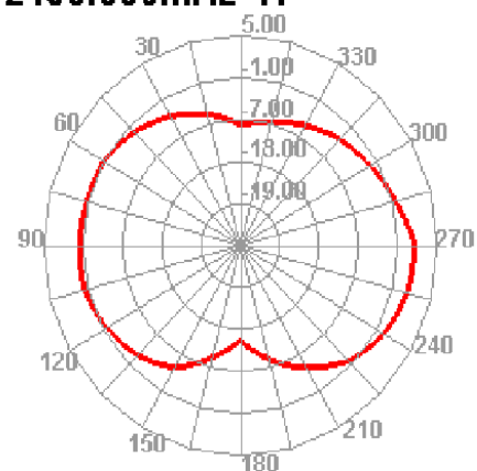
2450.000MHz H
