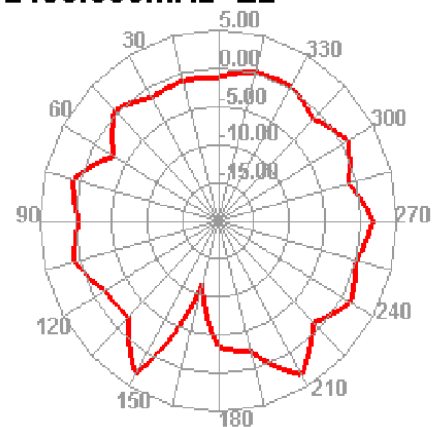
2450.000MHz E2
