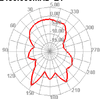
2400.000MHz E1
