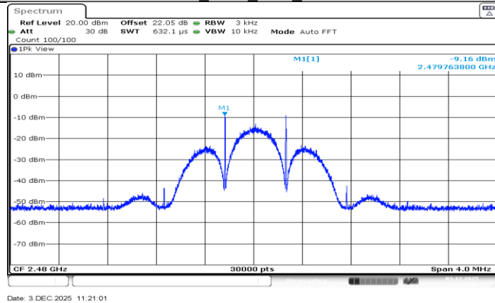
BLE_125K_Ant1_2480
