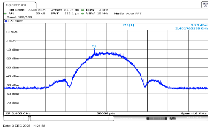
BLE_500K_Ant1_2402
