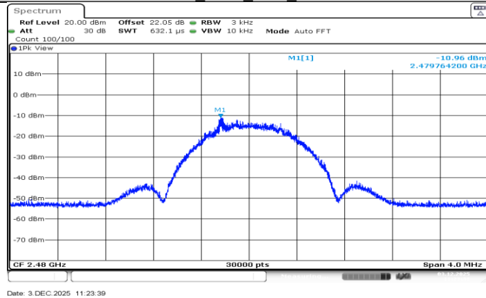
BLE_500K_Ant1_2480
