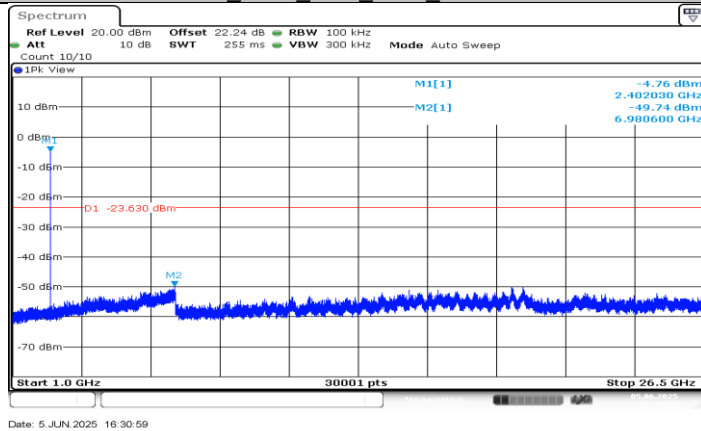
BLE_500K Ant1_2402_1000~26500
