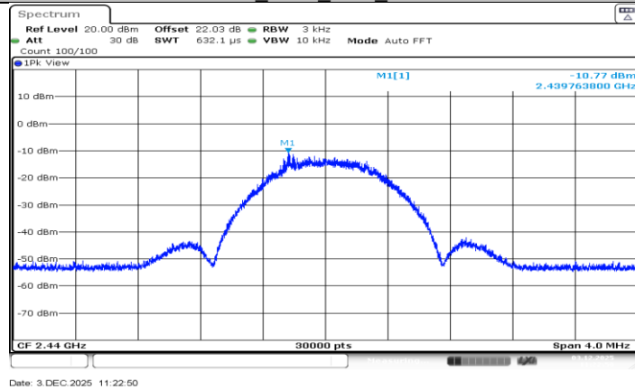
BLE_500K_Ant1_2440
