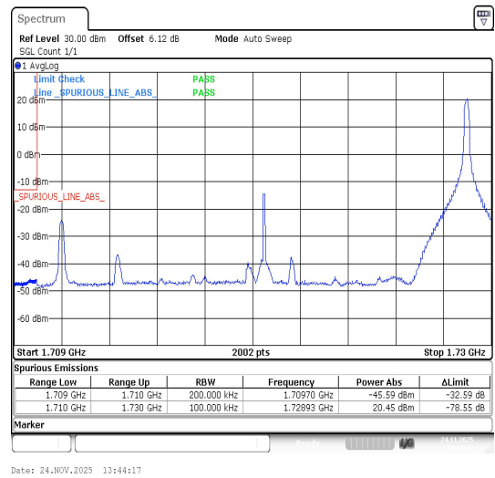
Band66-20MHz-QPSK-132072-1RB#99-PASS
