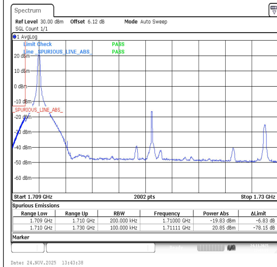
Band66-20MHz-QPSK-132072-1RB#0-PASS
