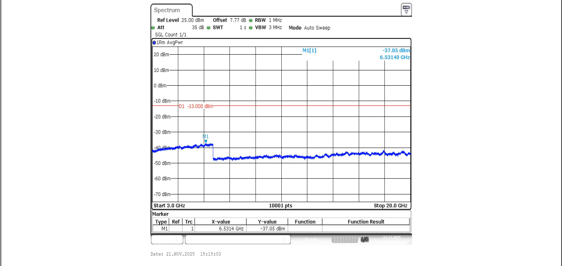
Band2-9400-3-3000~20000MHz-PASS
